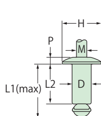
座屈側形状
