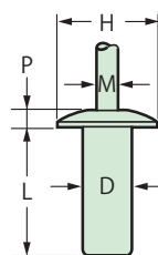
丸頭(D)
