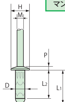
丸頭(D)
