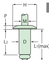
丸頭 (D)
